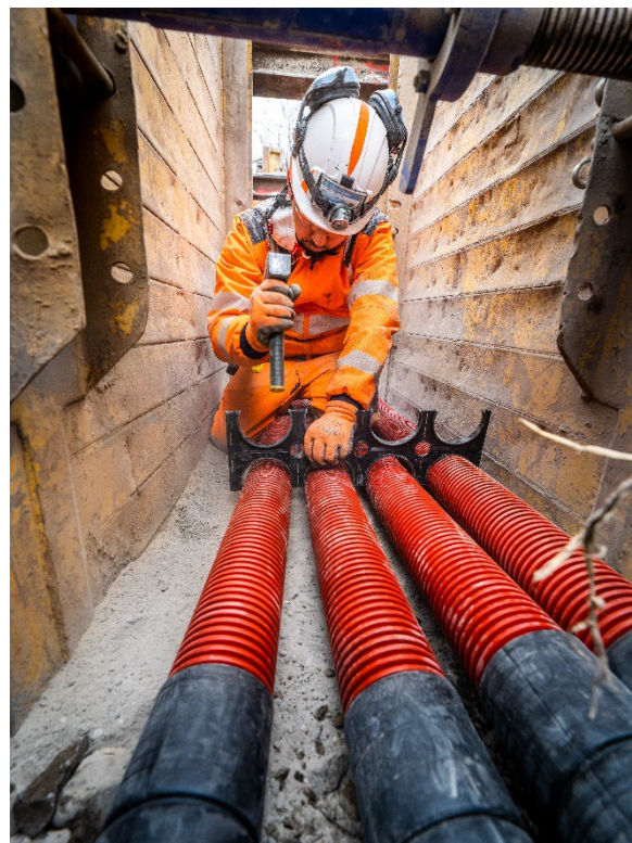
DÉVOIEMENT DE RÉSEAUX, GARE DE VILLIERS-SUR-MARNE (77)
