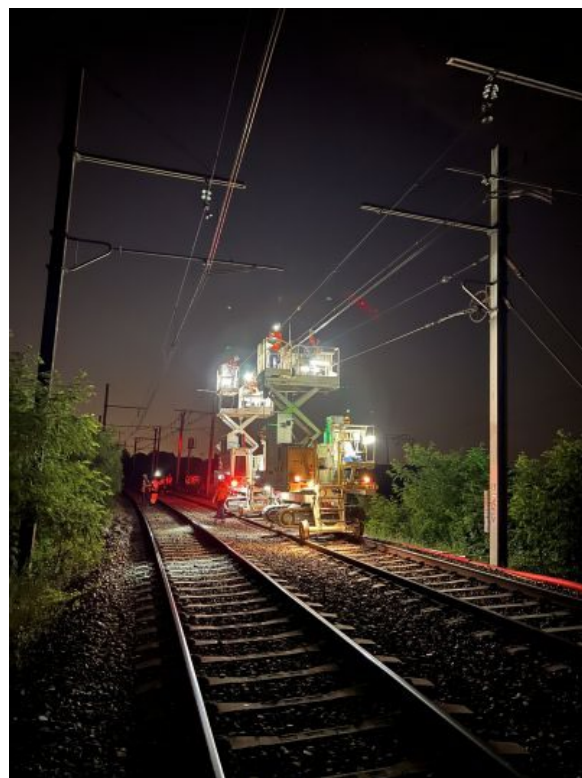
RENFORCEMENT DE CATÉNAIRES SUR LA LIGNE DU RER D
